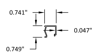
41 SMI GLASS STOP 6063-T5
