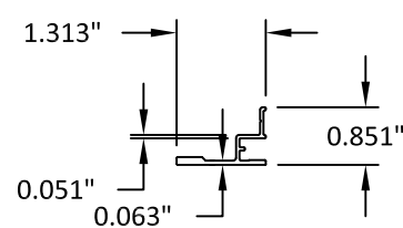
10 ADAPTOR 6063-T5
