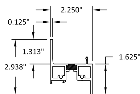
5 MULLION 6063-T5
