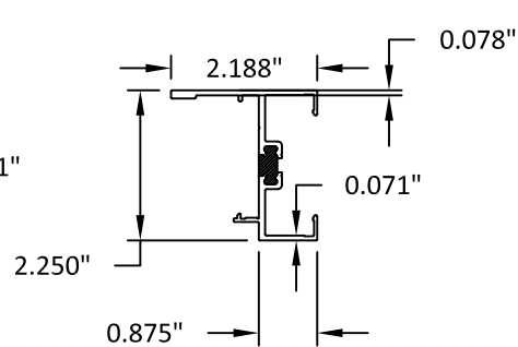
2 FRAME JAMB 6063-T5
