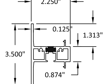
6 MULLION 6063-T5
