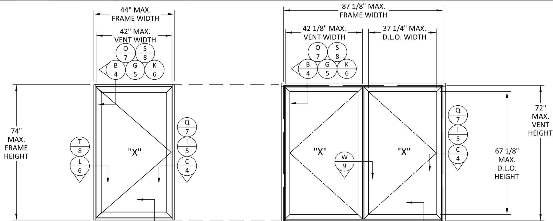
ELEVATION
