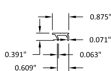
19 LOCK BAR BASE 6063-T5
